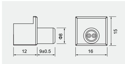
Integral end cap
